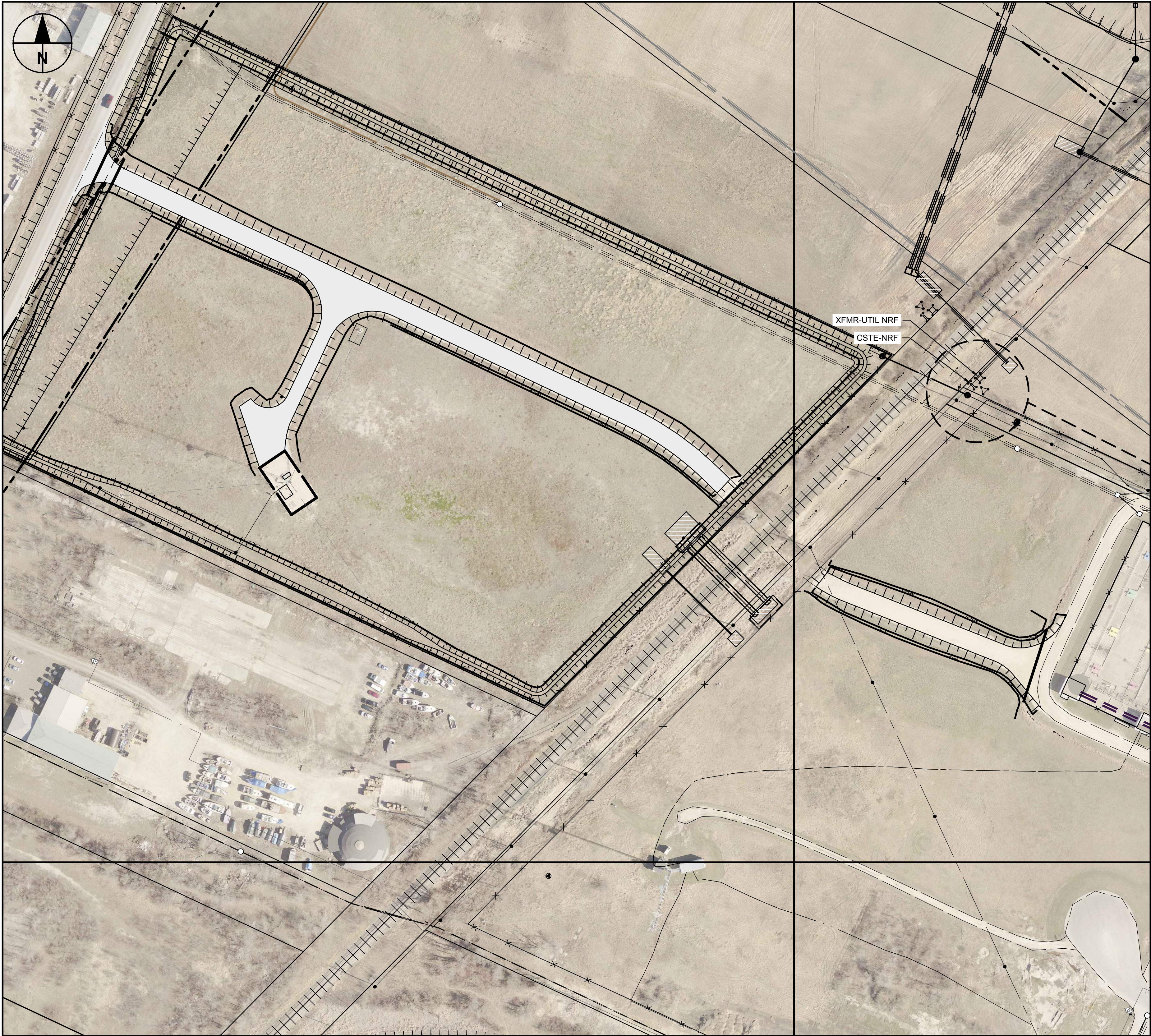
SITE PLAN SCALE: 1:1000
